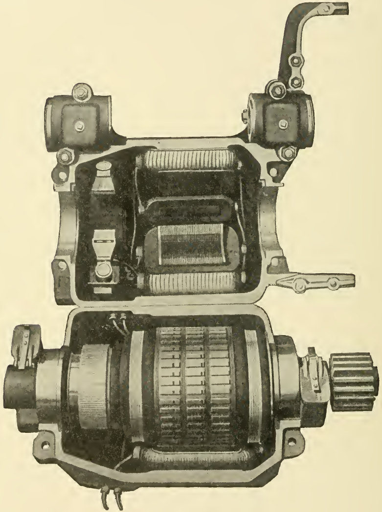
Fig. 44. Allis-Chalmers Inter-pole Motor
